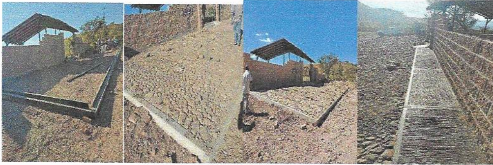
CONSTRUCCION DE LINEA DE DRENAJE Y EMPEDRADO AHOGADO EN CONCRETO EN CALLE ROMERO DE LA LOCALIDAD DE SAN PEDRO MUNICIPIO DE ATENGO, JALISCO MONTO TOTAL= $1, 194,598.23
